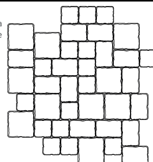
POSA "ALLA ROMANA" questa posa prevede uno schema casuale, prestare attenzione alle quantità (pz/m 2 ) dei masselli utilizzati
